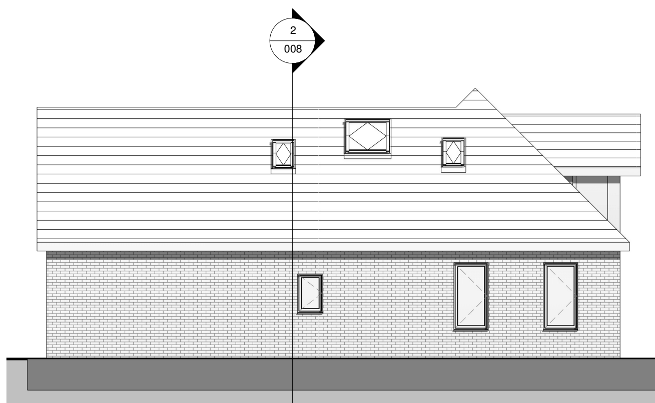
Right Elevation
